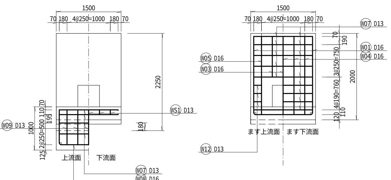
正面图
