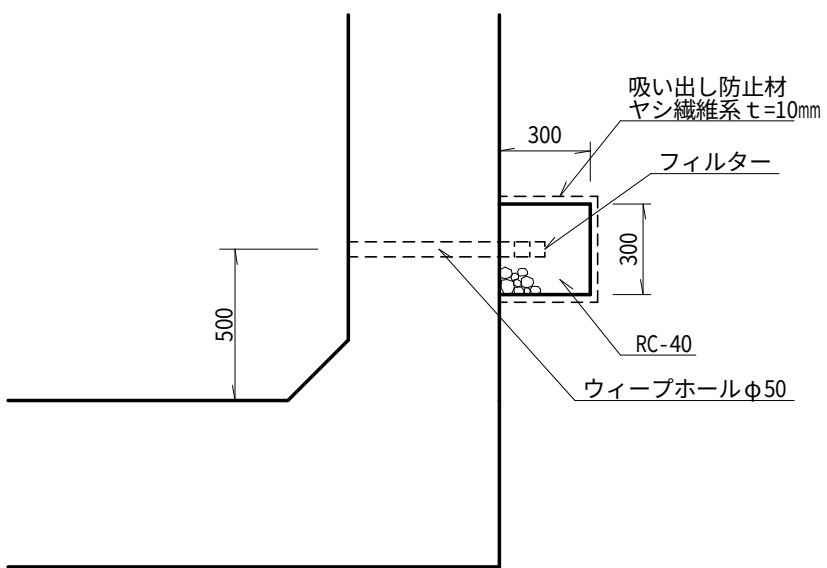
サイドドレーン詳細図 S=NON
