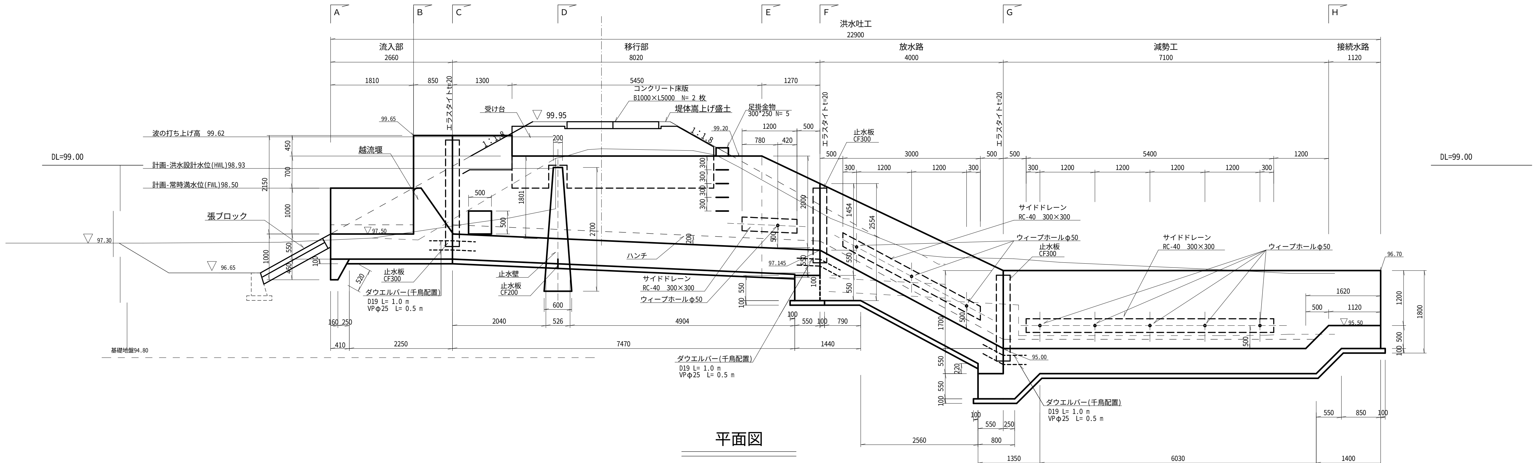
洪水吐構造図 S=1:50 側面図
