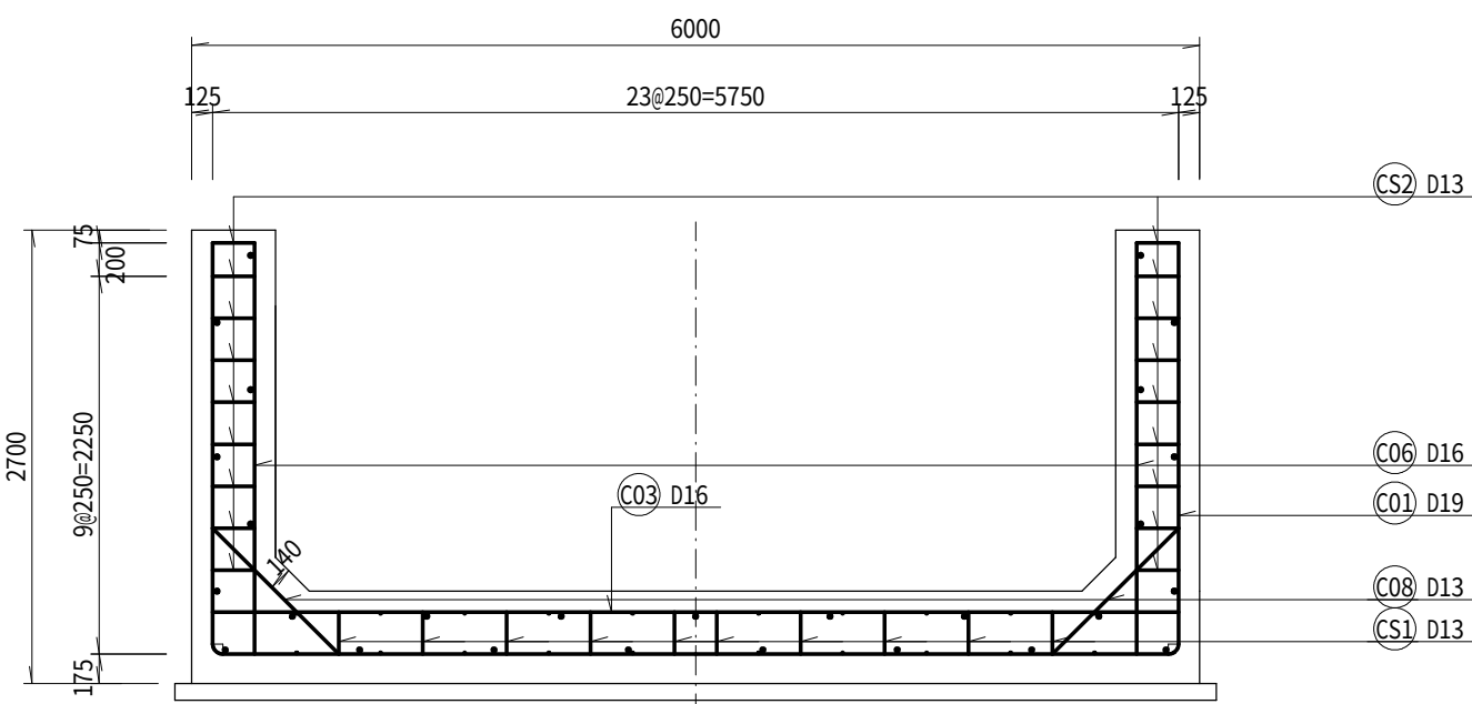
正面図 C-C'
