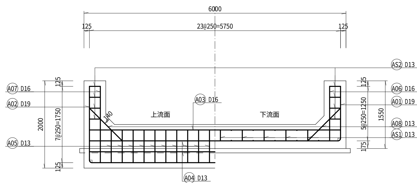
B-B'
