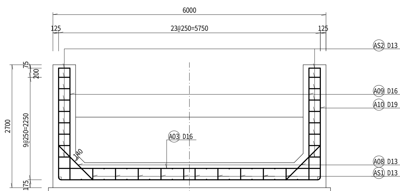
B-B'
