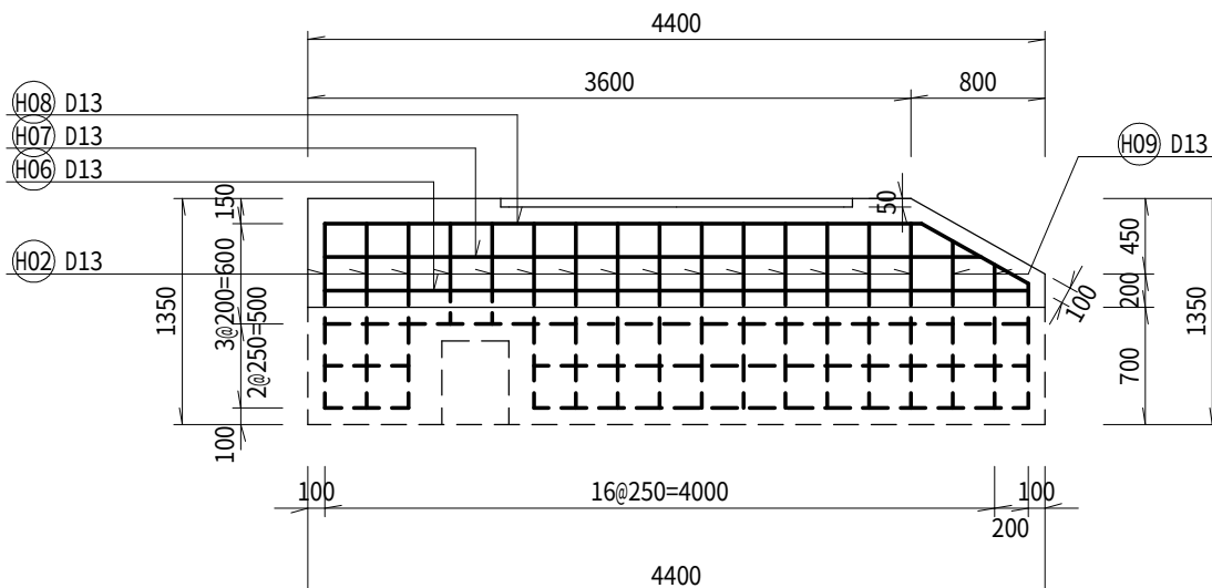
平面図 上側
