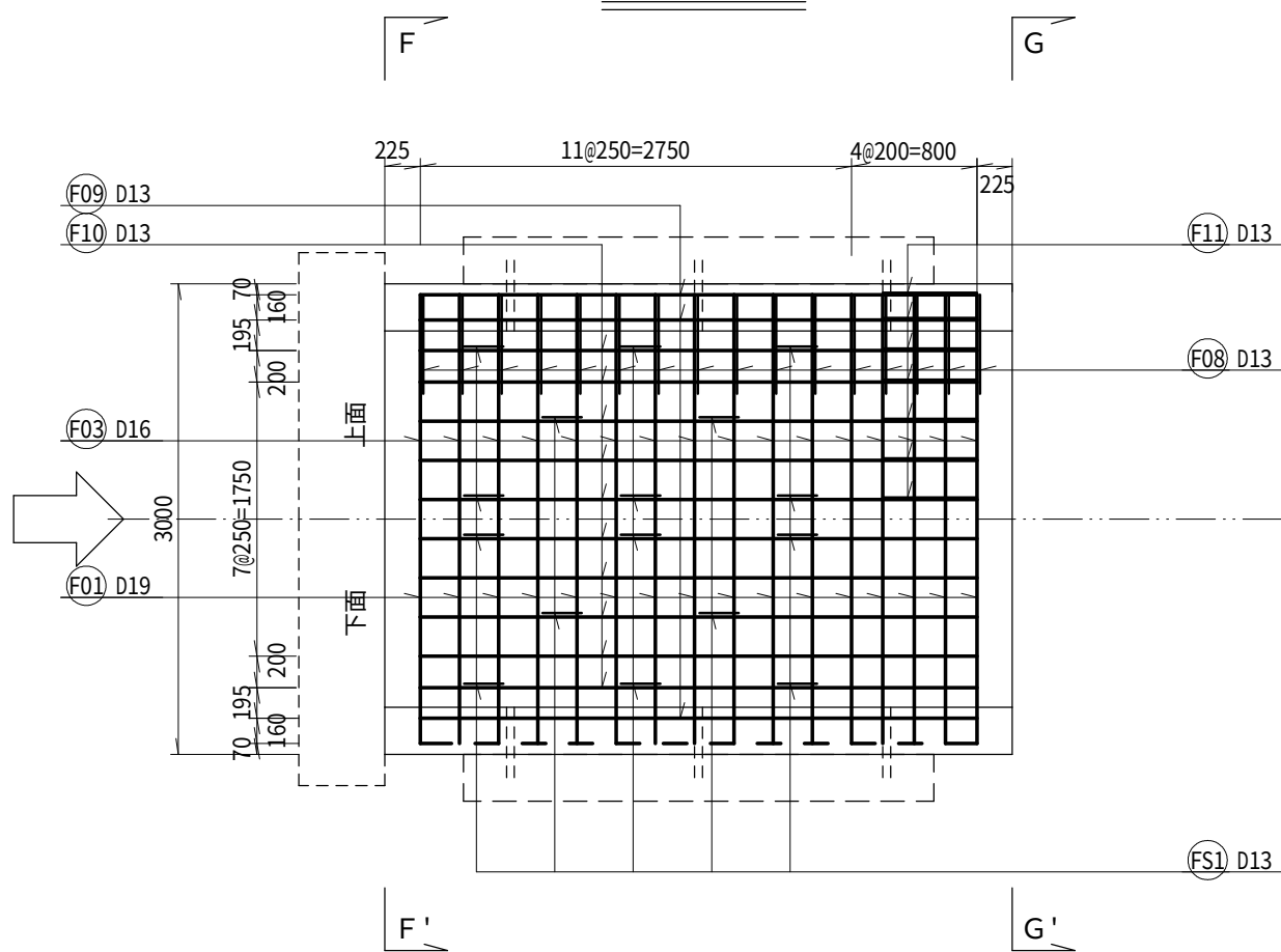
平面図
