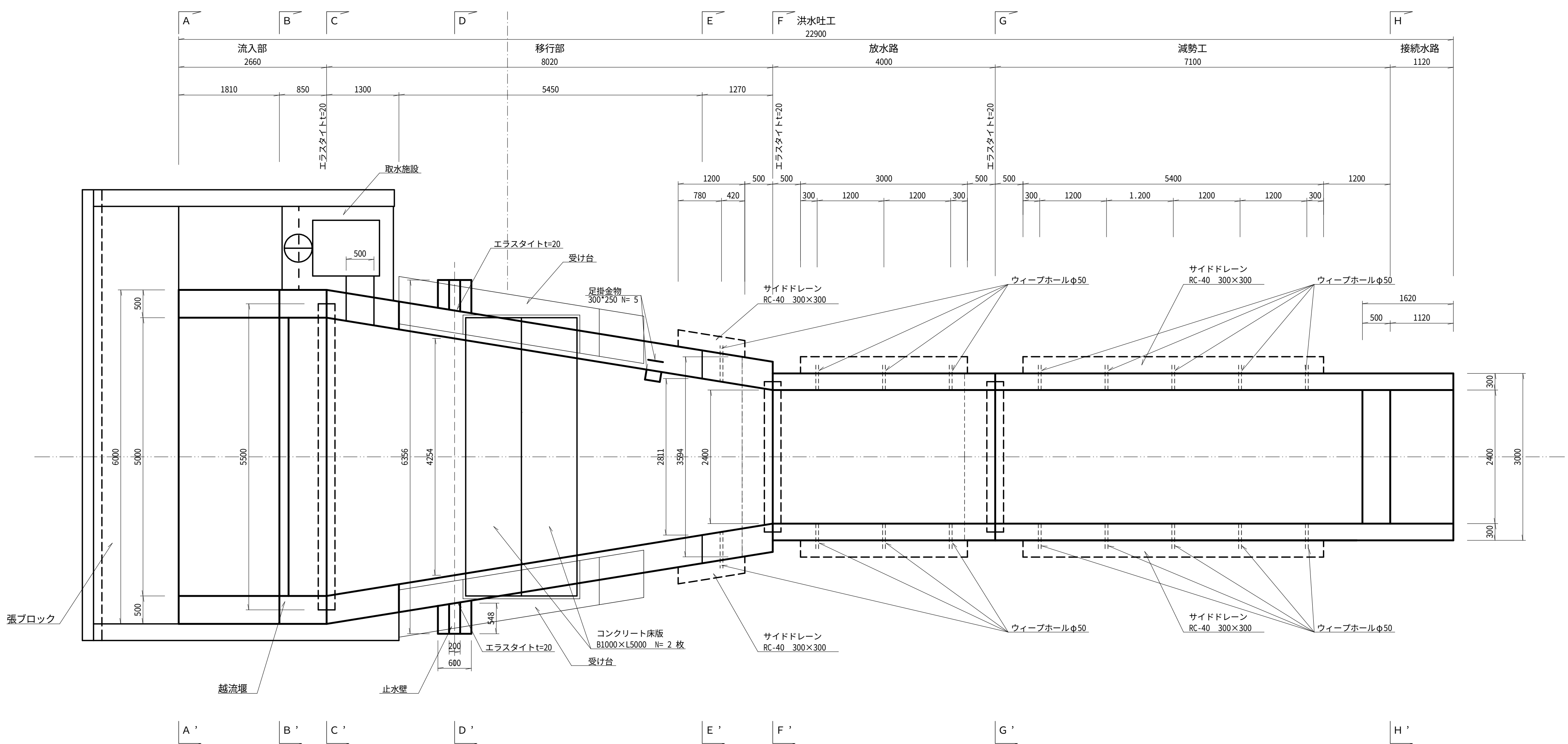
平面図
