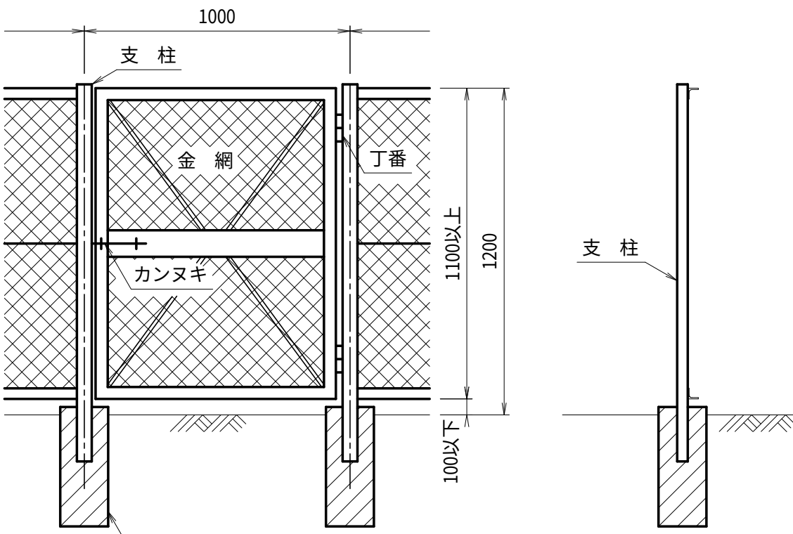
ネットフェンス扉、片開1200型 S=1：20 亜鉛メッキ製
