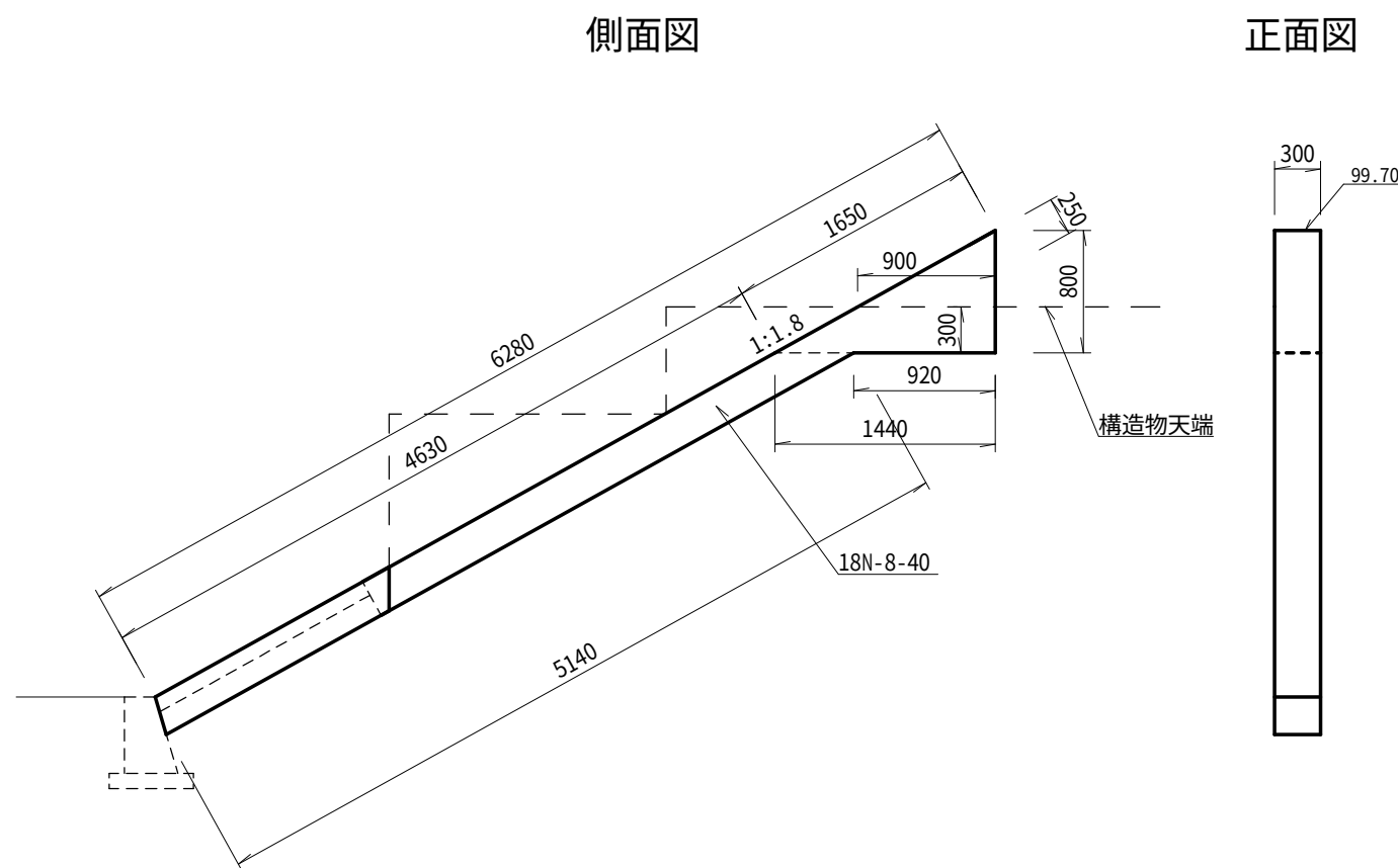
2型小口止め
