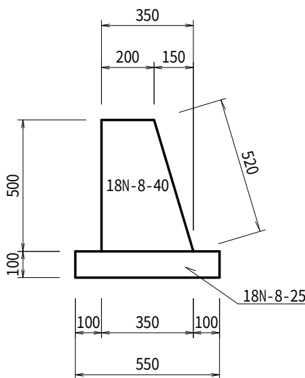
基礎コンクリート S=1：20
