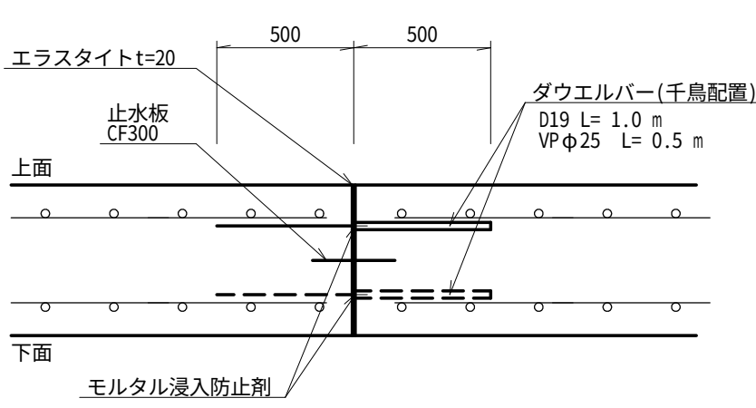
継ぎ目工詳細図 S=NON
