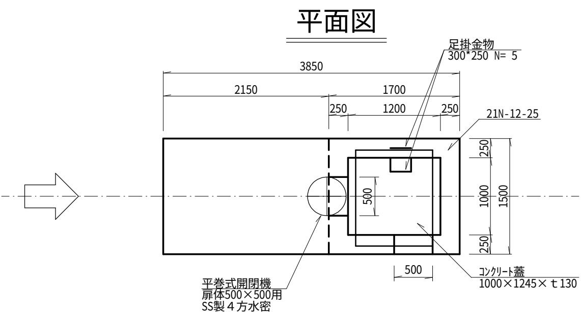
取水施設工 S=1:50
