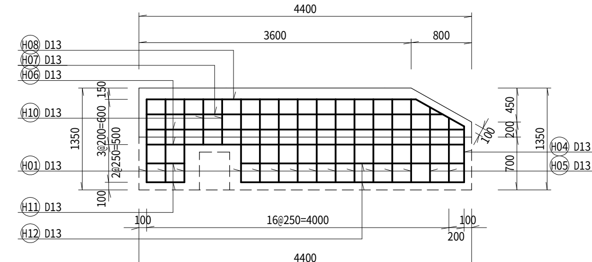
側面図 内側
