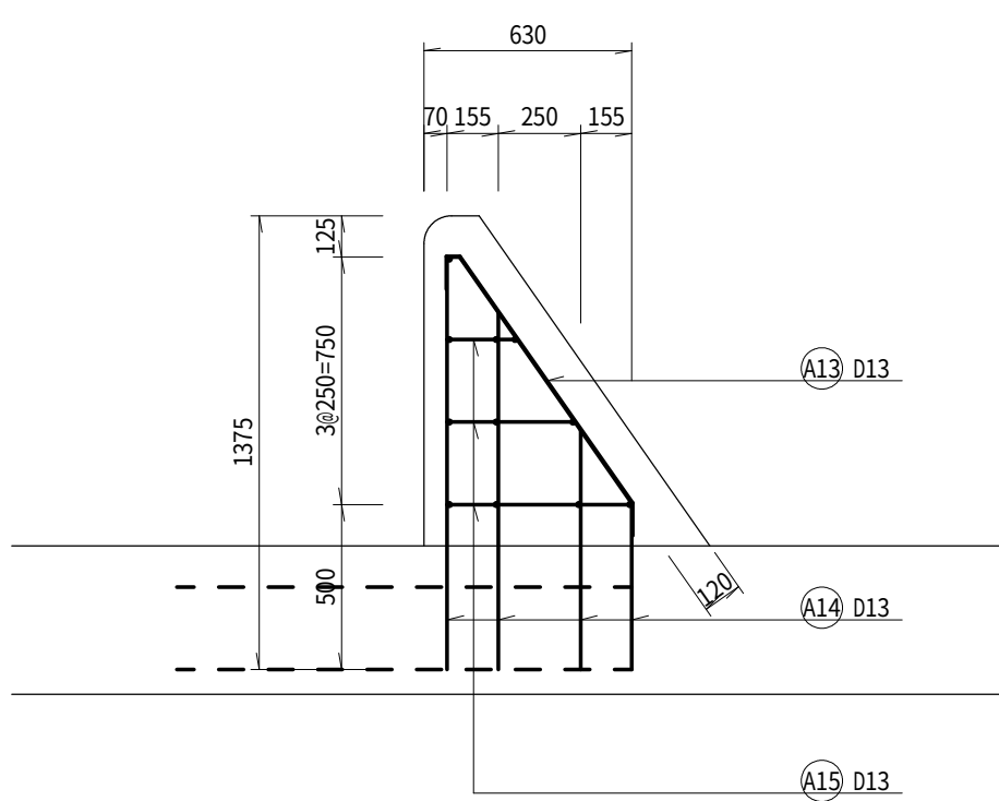
越流堰詳細図 S=1 : 25
