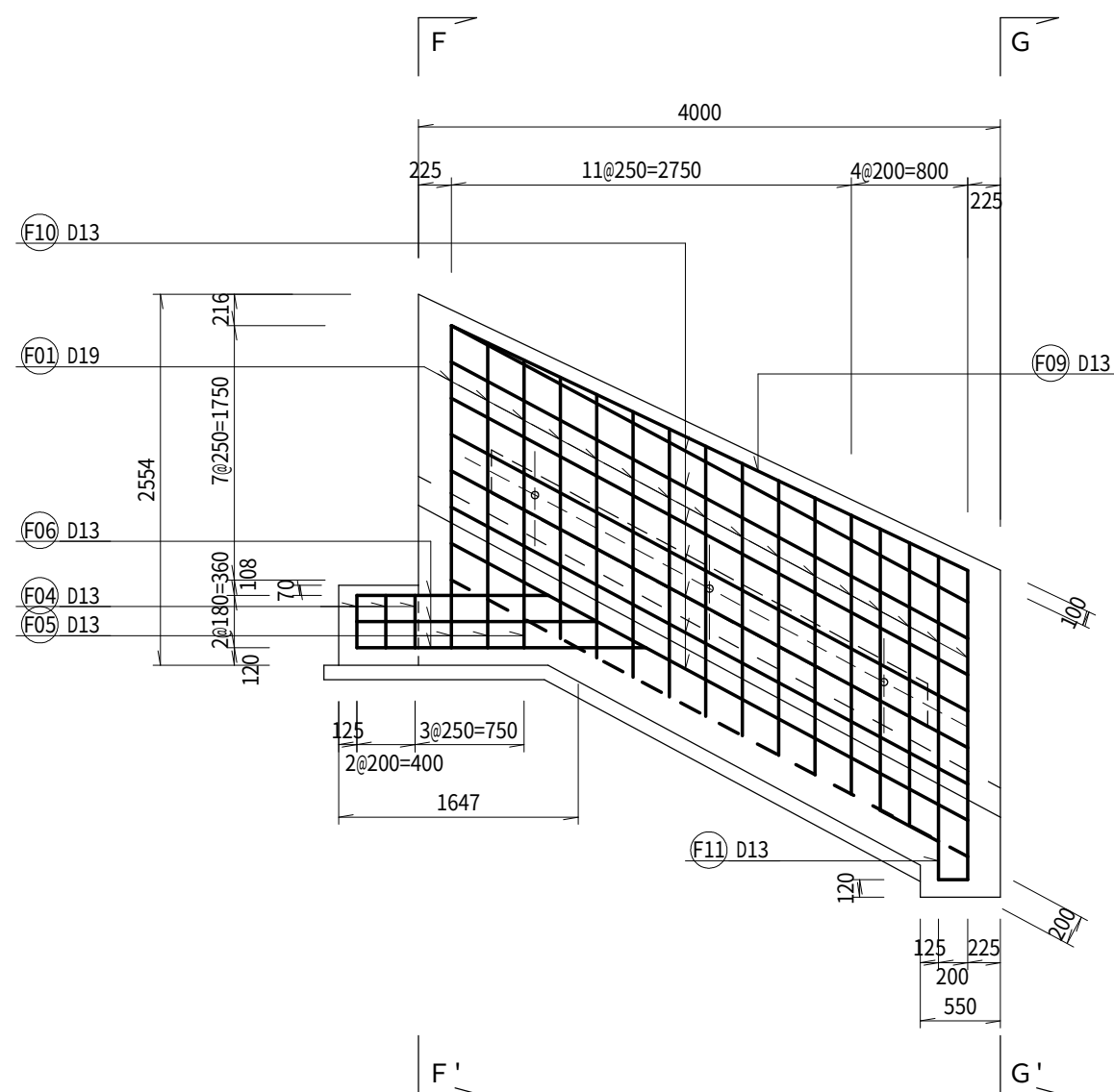
側面図 内側
