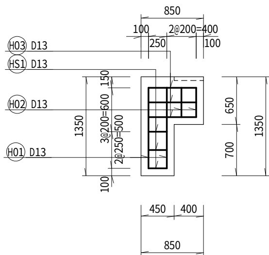
正面図 上流側
