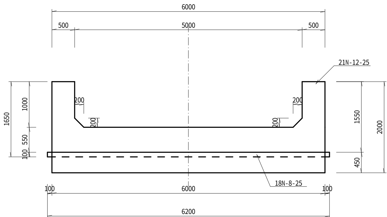
B-B'
