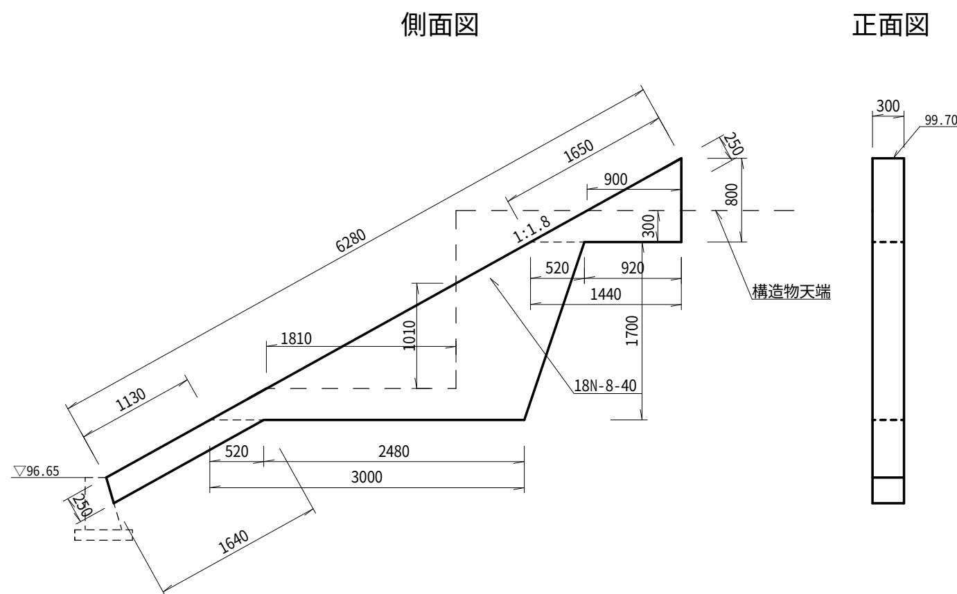
1型小口止め
