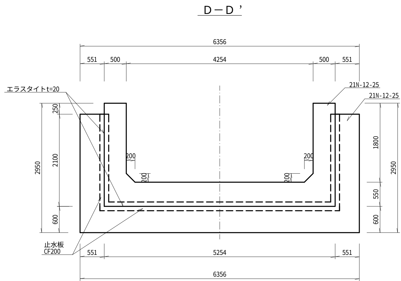
止水壁詳細図 S=NON
