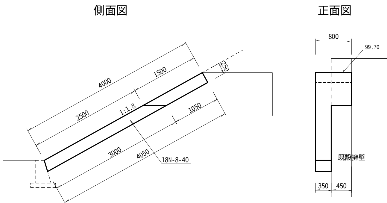
3型小口止め
