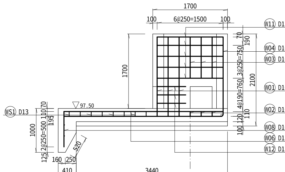
側面図 右側
