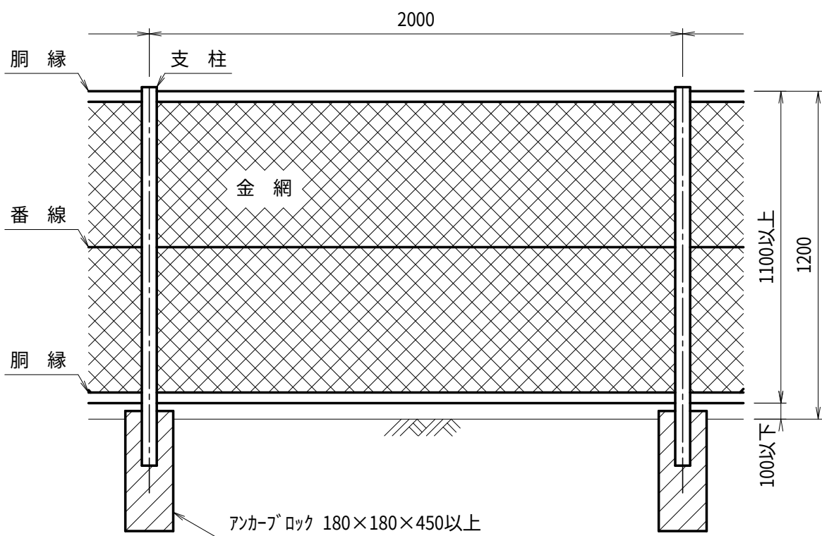
ネットフェンス1200型 S=1：20 亜鉛メッキ製
