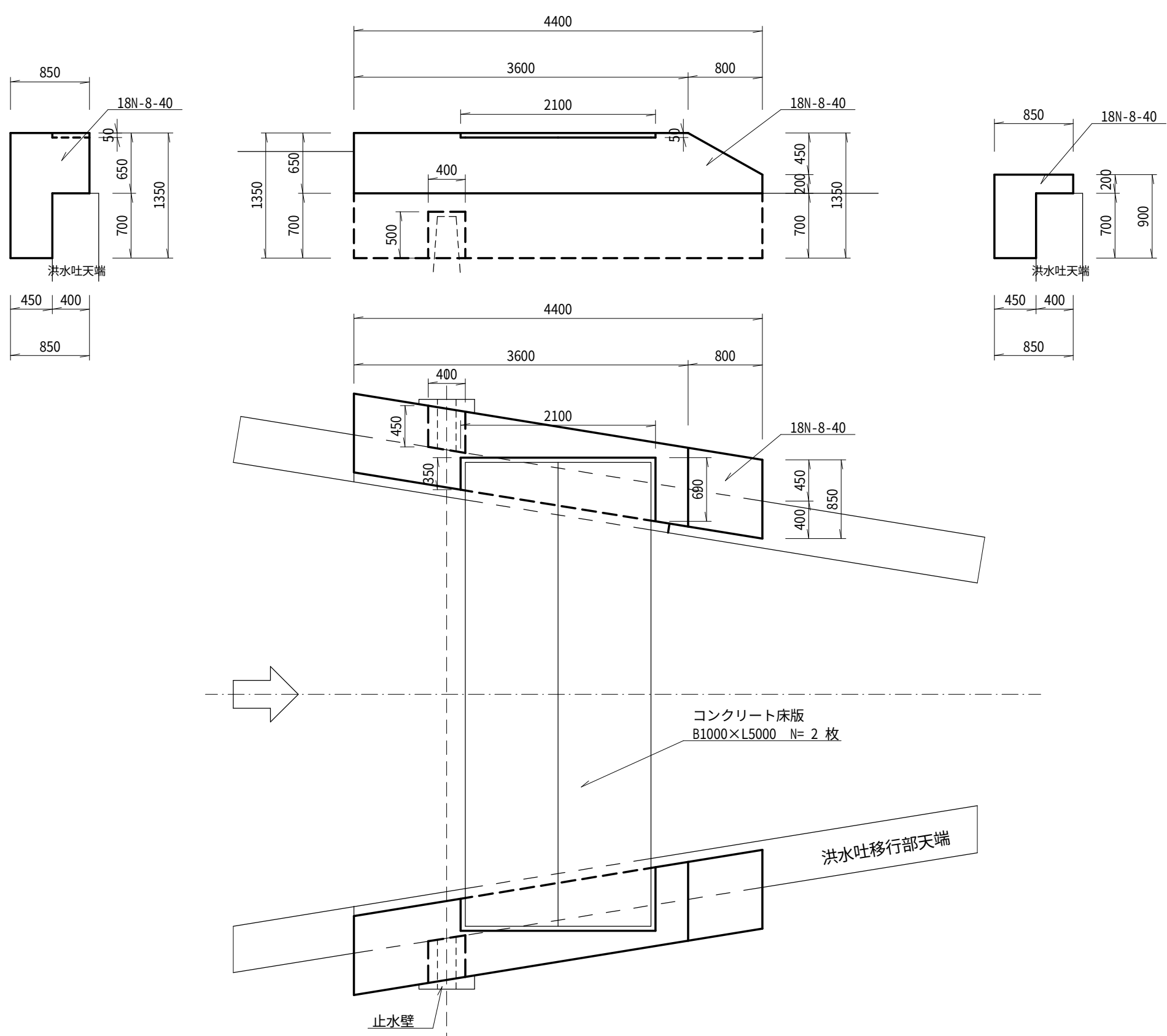
受け台 S=1:50
