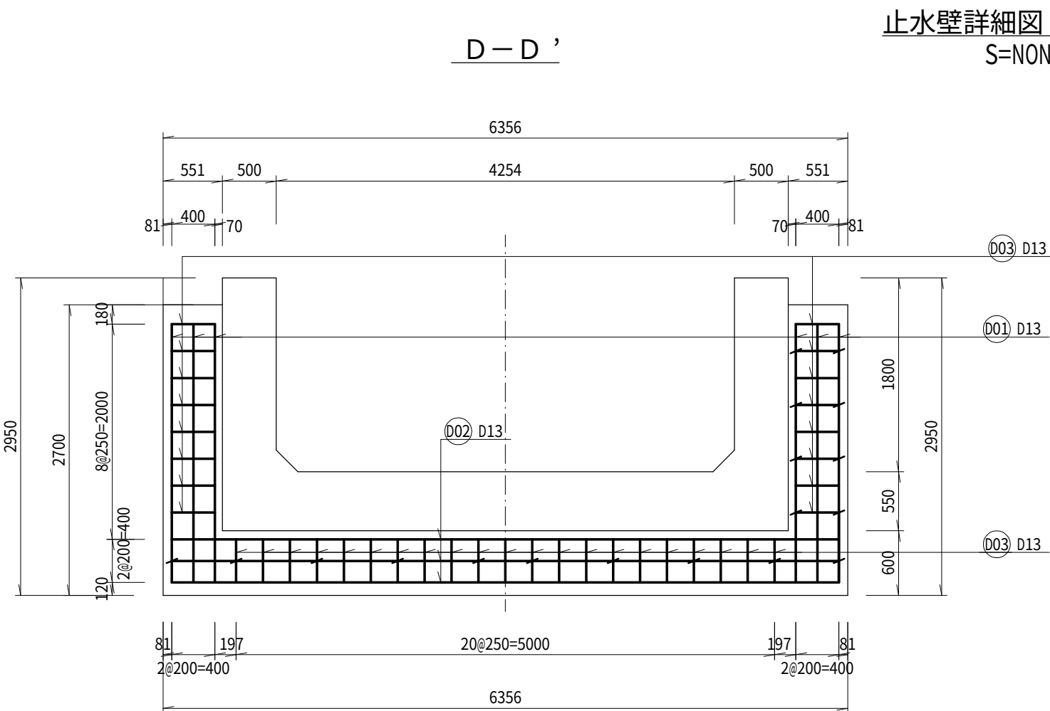
移行部 S=1 : 50
