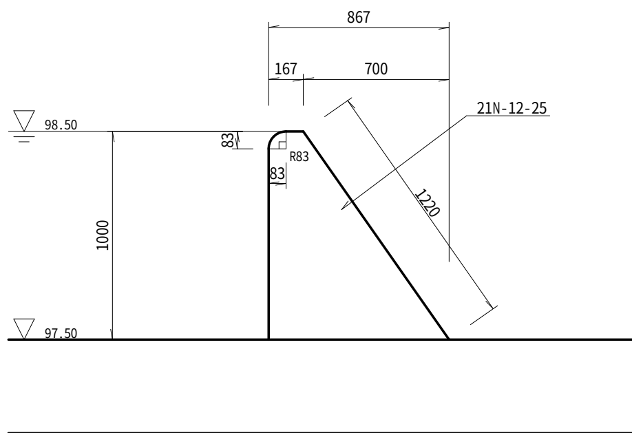
越流堰詳細図 S=NON
