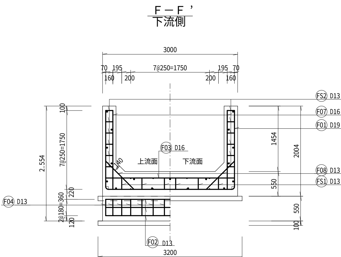
正面図
