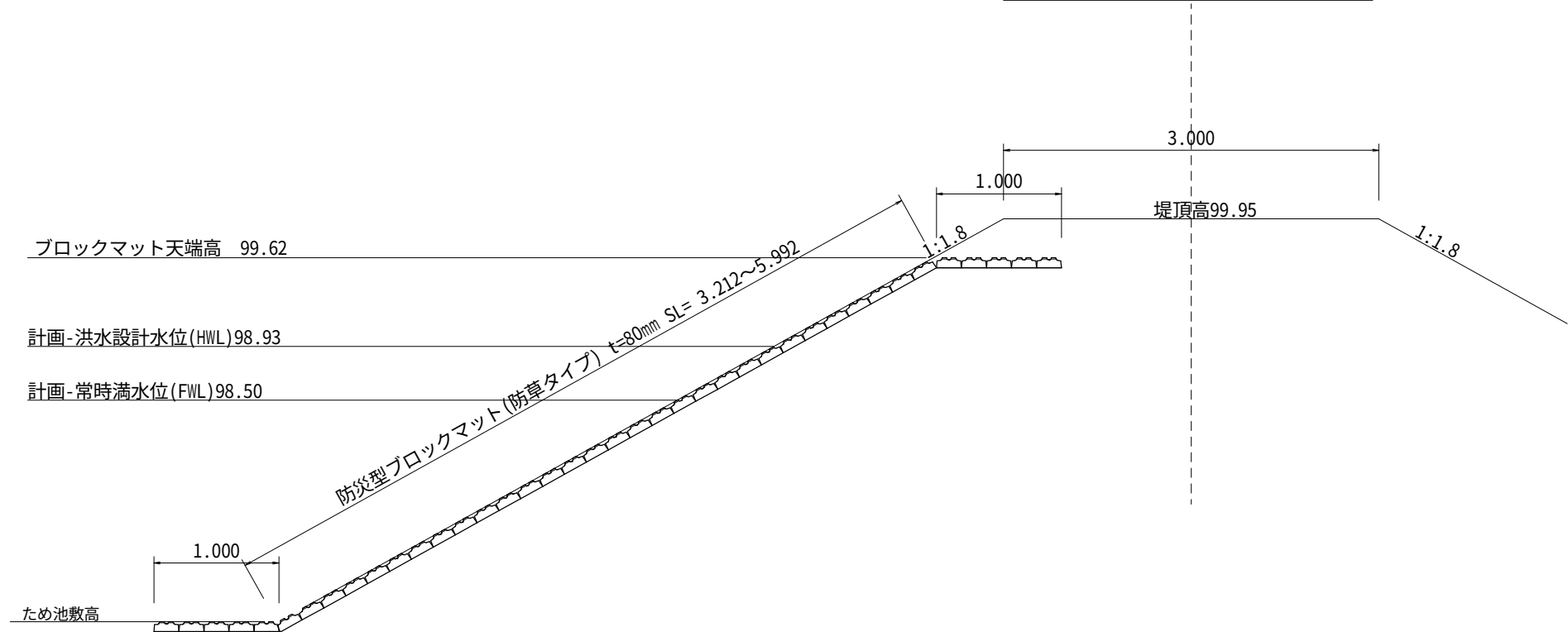
標準断面図 S=1：50
