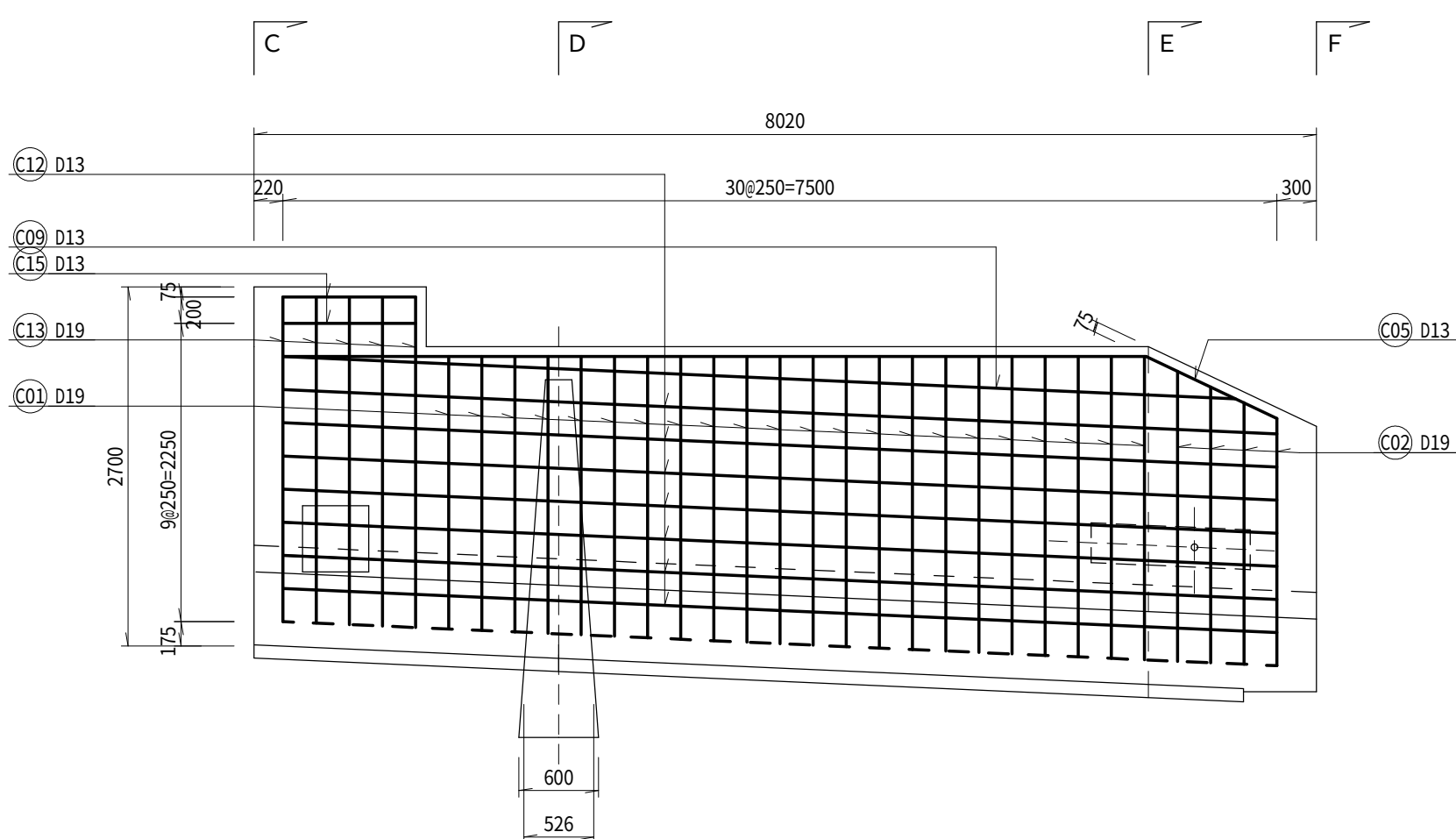
側面図 内側
