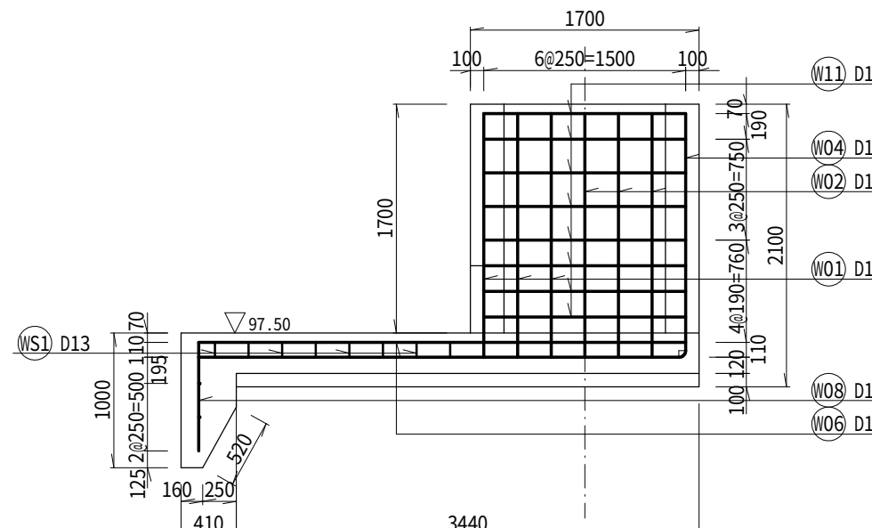
側面図 左側
