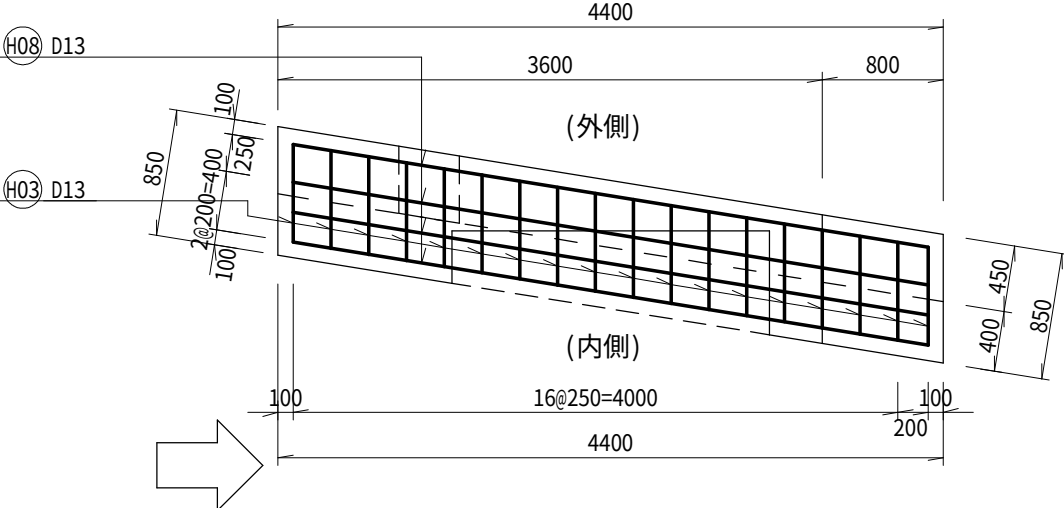
平面図 上側
