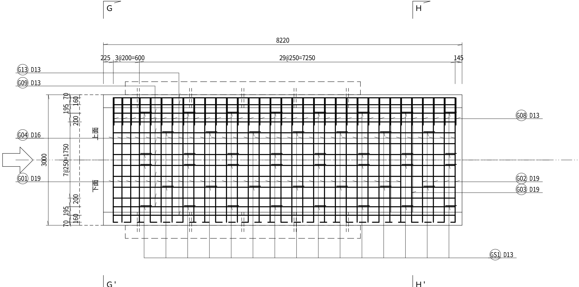
平面图
