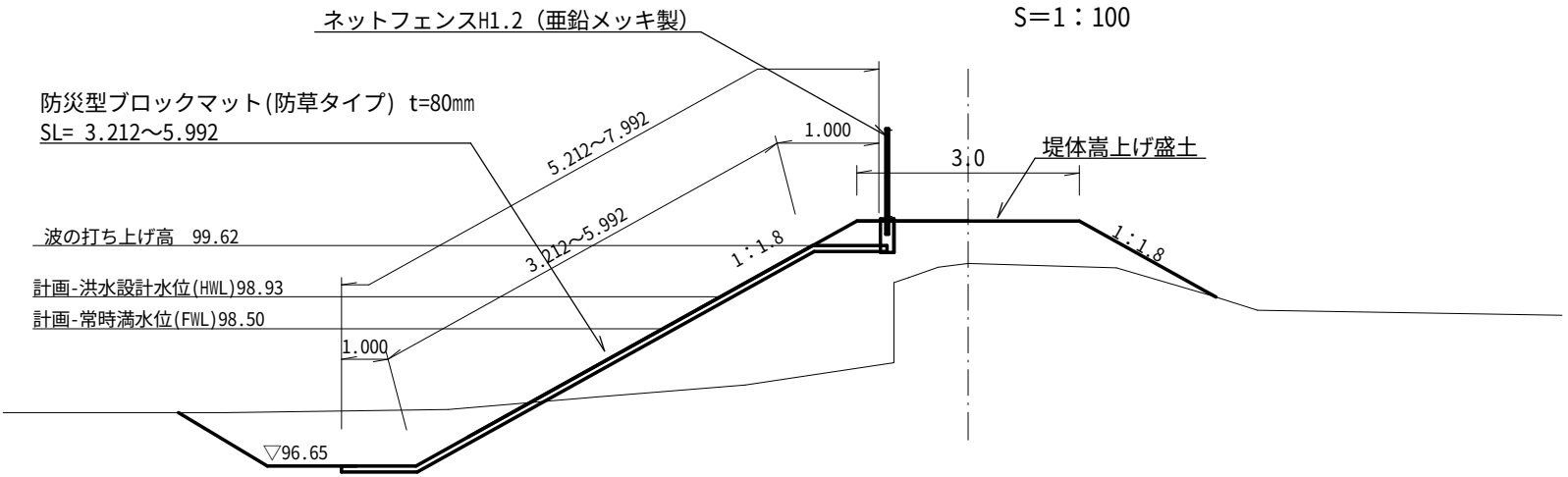
標準断面図
