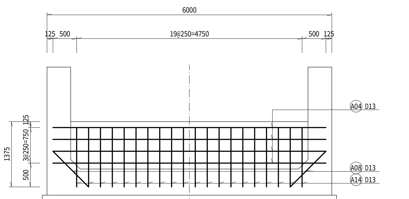
B-B' 越流堰
