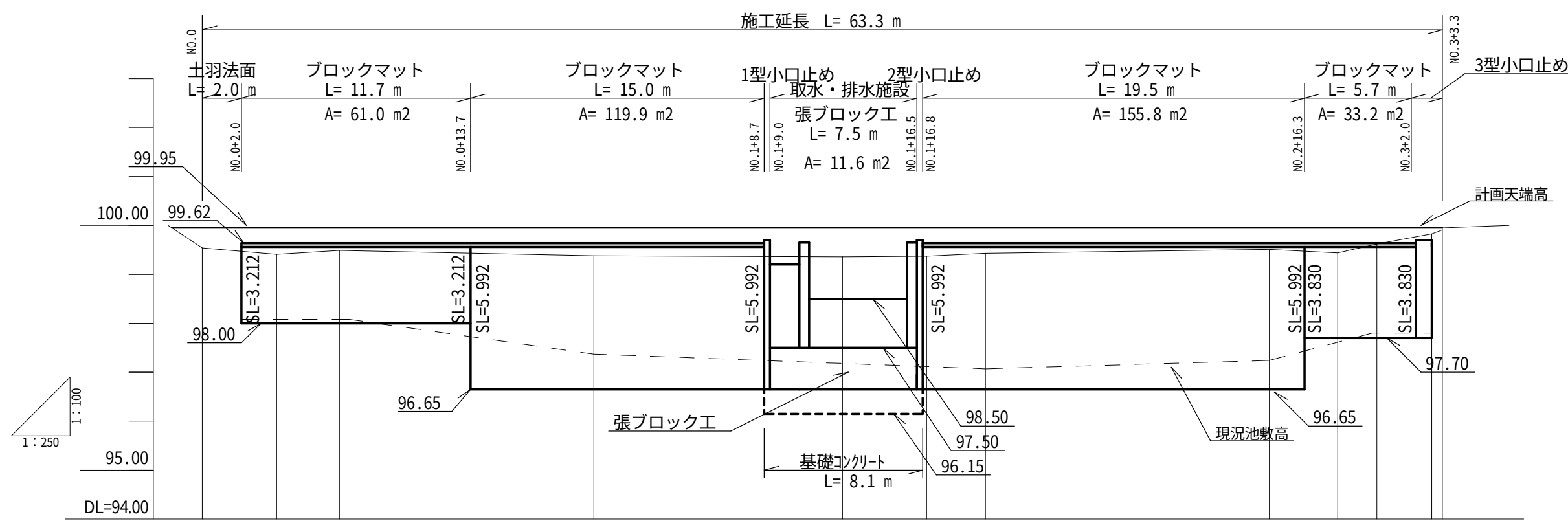
縦断図 SV=1：100 SH=1：250
