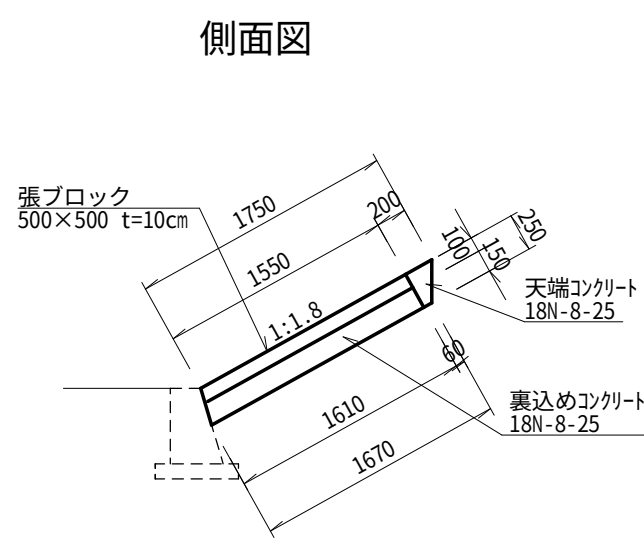
張ブロック工 S=1：50
