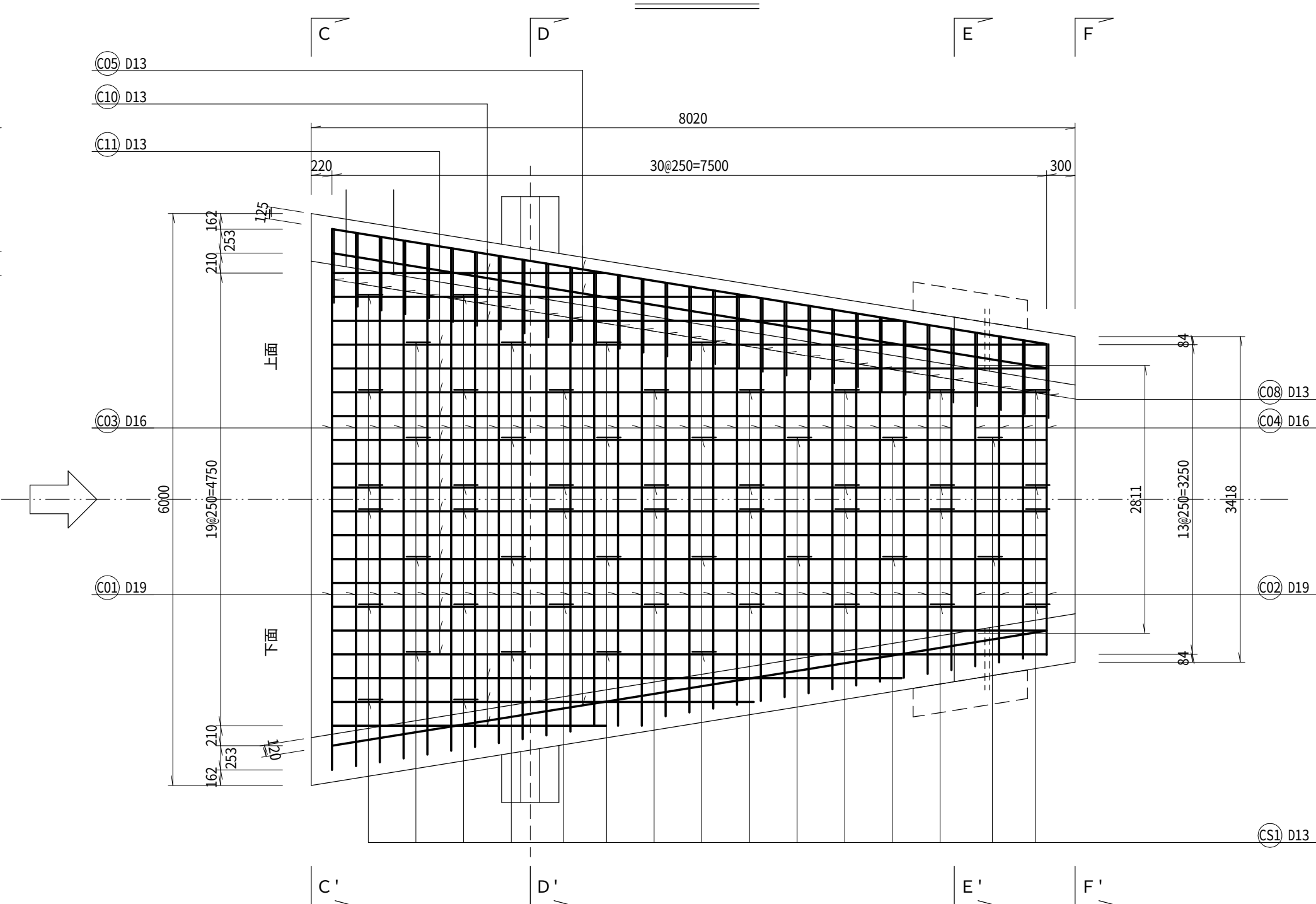
平面図
