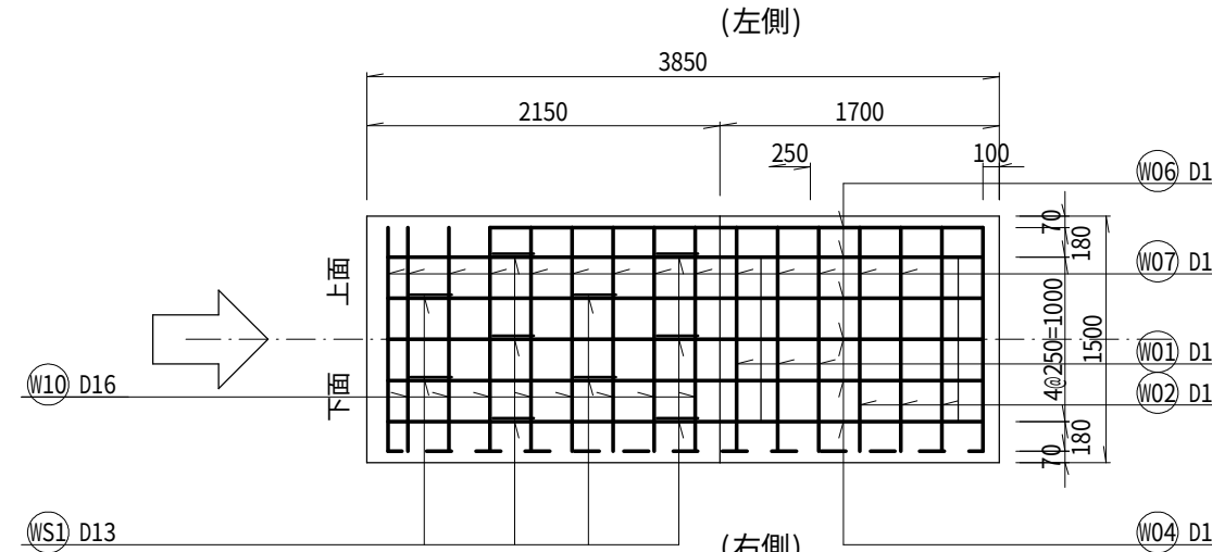
側面図 右側
