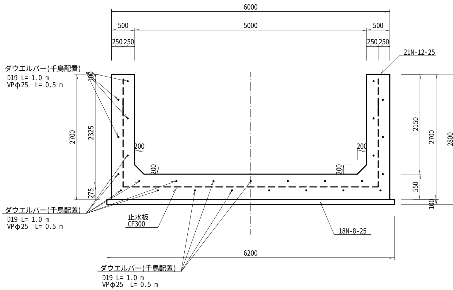
C=C' 上流側
