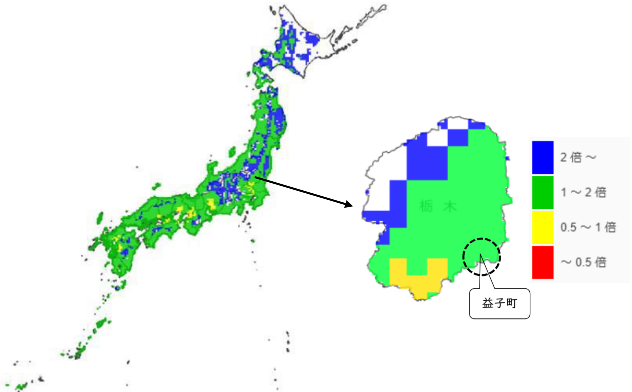
現行の移植日と栽培管理を想定した場合の粗玄米収量の変化
